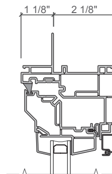
3-1/4-in. nail fin frame
