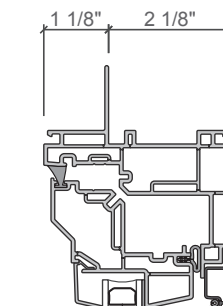
3-1/4-in. nail fin frame
